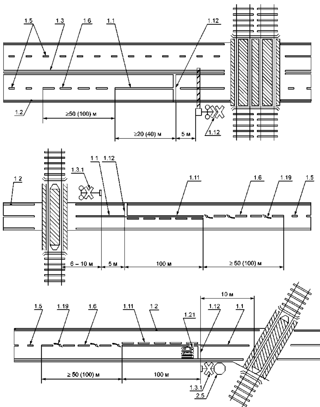
Рисунок В.18 - Примеры разметки участка дороги на подъезде
