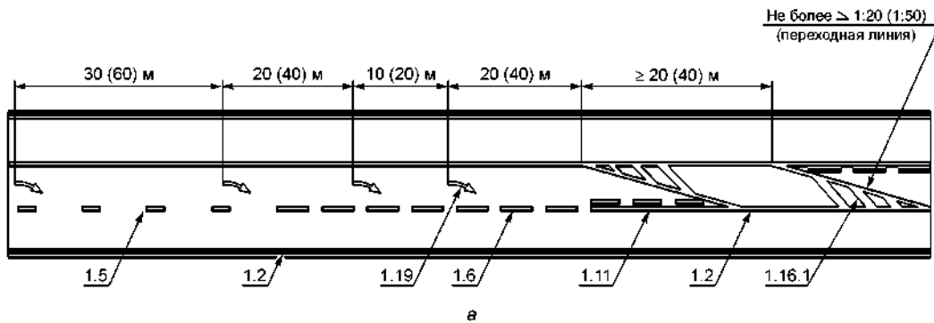
Рисунок В.7 - Пример нанесения разметки перед нерегулируемым перекрестком с ограниченной видимостью
